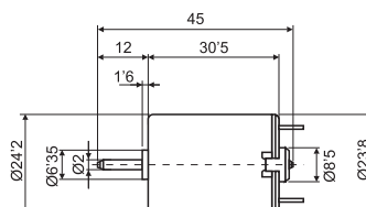
70.541 MOTOR MINIATURA
