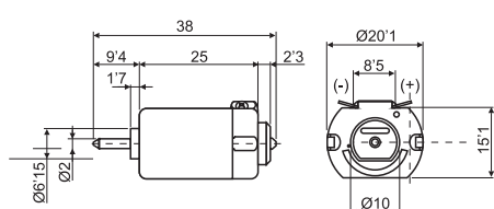
70.501 MOTOR MINIATURA
