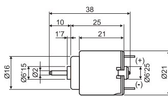
70.521 MOTOR MINIATURA
