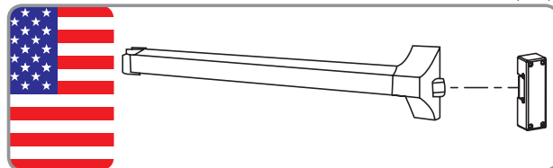
MONTAJE CON BARRA ANTIPÁNICO ESTÁNDAR AMERICANO (82P)
