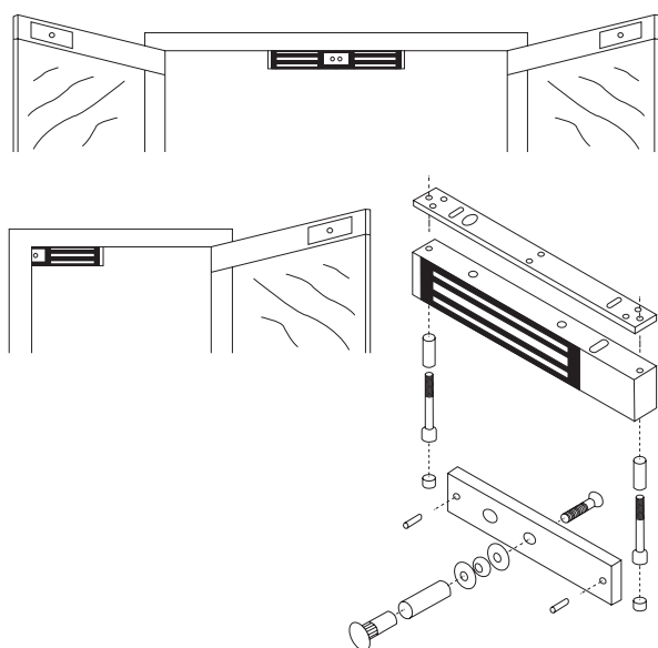
Esquema Sobreponer
