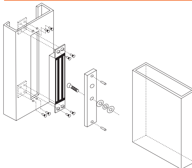
Esquema Empotrar
