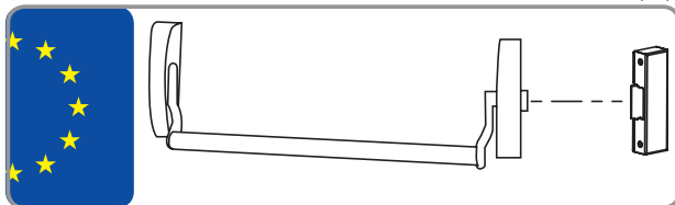
MONTAJE CON BARRA ANTIPÁNICO ESTÁNDAR EUROPEO (82)
